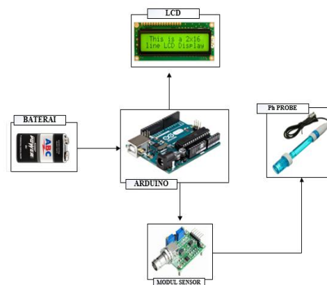
Gambar 6 Diagram Blok Sistem
