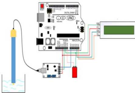
Gambar 7 Wiring Diagram Perancangan
