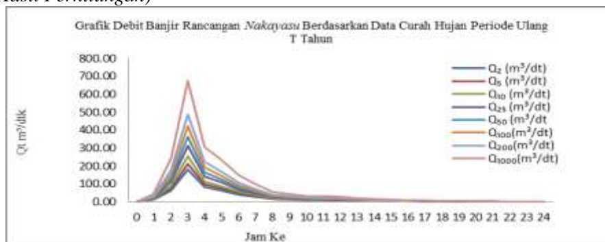
Gambar 1 Debit Banjir Rancangan Nakayasu Berdasarkan Data Curah Hujan Periode Ulang T Tahun
