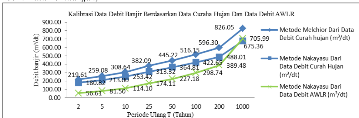
Gambar 3 Grafik Kalibrasi Data Debit Berdasarkan Data Curah Hujan Dan Data Debit AWLR
