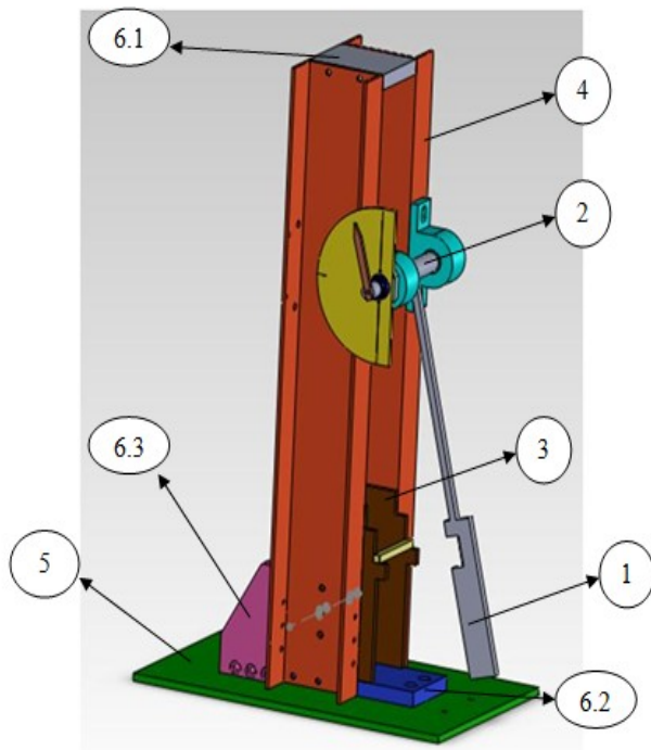
Gambar2. Komponen alat uji impact charpy untuk material plastik
