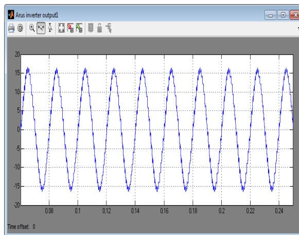
22. Bentuk gelombang keluaran arus inverter berupa sinusoidal-segitiga.
