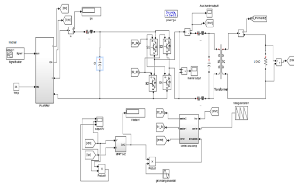
Gambar 16. Simulasi Model kontrol arus ramp comparison current control yang diterapkan pada inverter PLTS off grid
