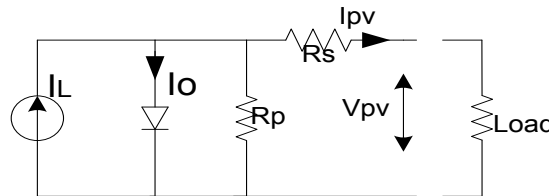
Gambar 5. Rangkaian ekuivalen sel PV [9]
