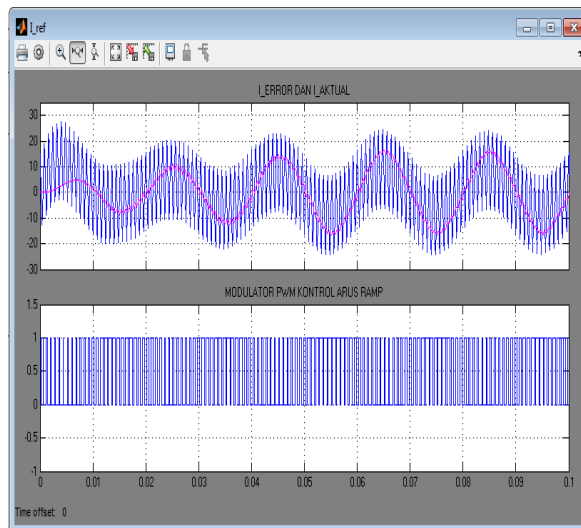
Gambar 21. Sinyal modulator PWM kontrol arus ramp dibentuk dari hasil perbandingan I error dengan I aktual
