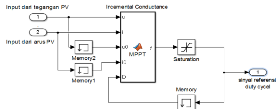
Gambar 14. Model algorithma MPPT dengan metode incremental conductance
