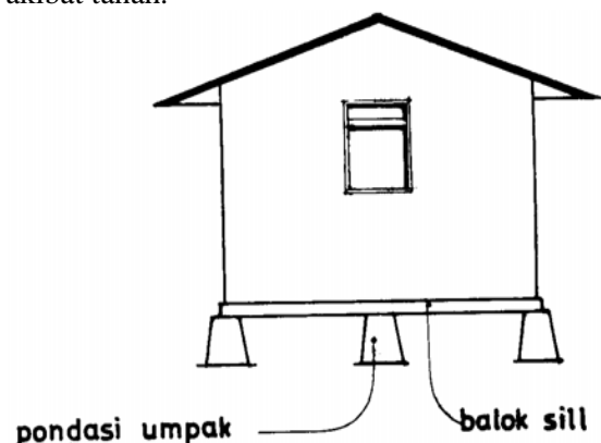
Gambar. 2 Pondasi umpak pada rumah sederhana [13].
