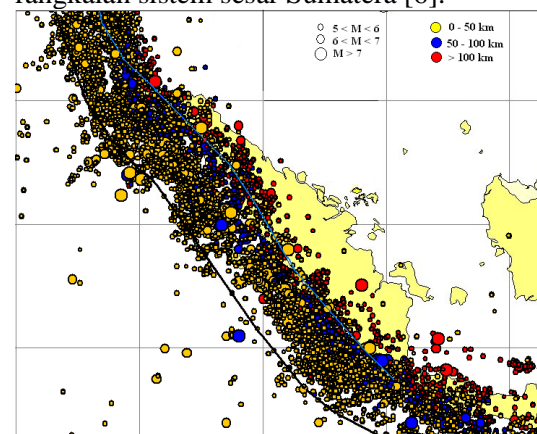
Gambar 1. Sebaran kegempaan di wilayah Sumatera [7].
