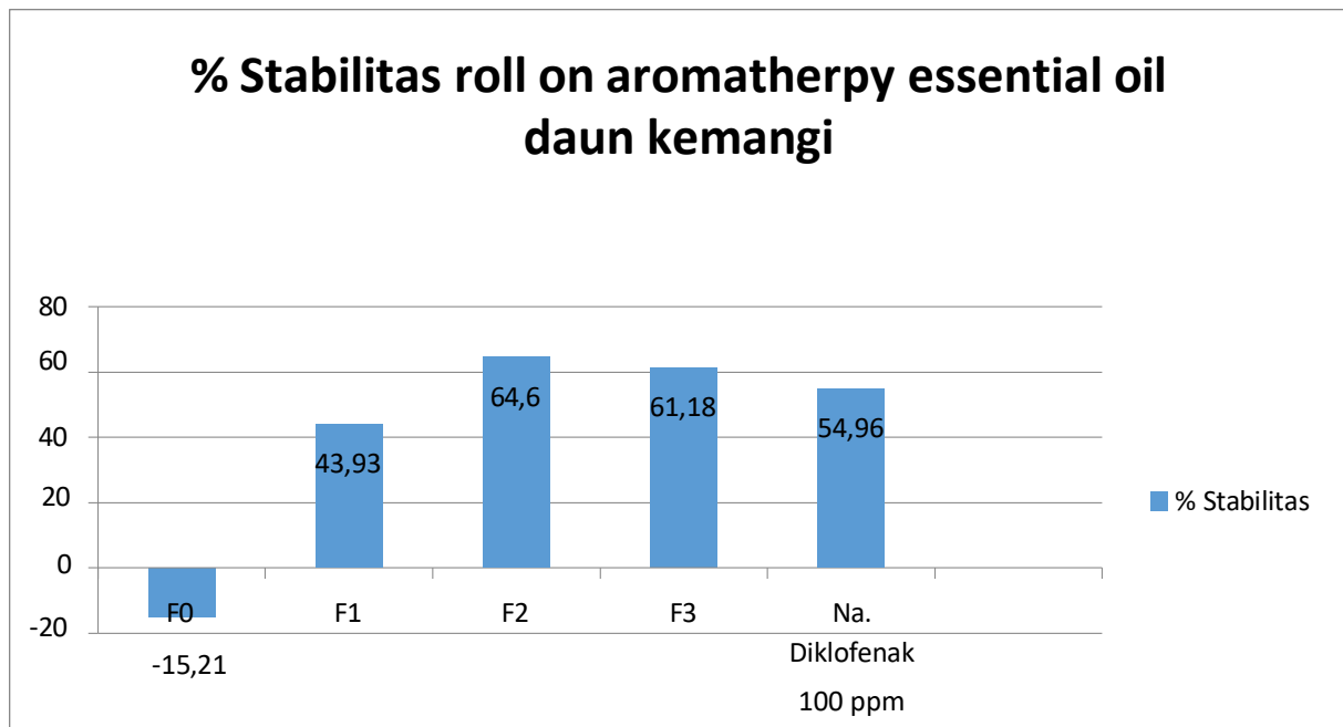
Gambar 5. Grafik Hasil Uji Stabilisasi Membrane Eritrosit Dari Roll On Aromatherapy Essential Oil Daun
